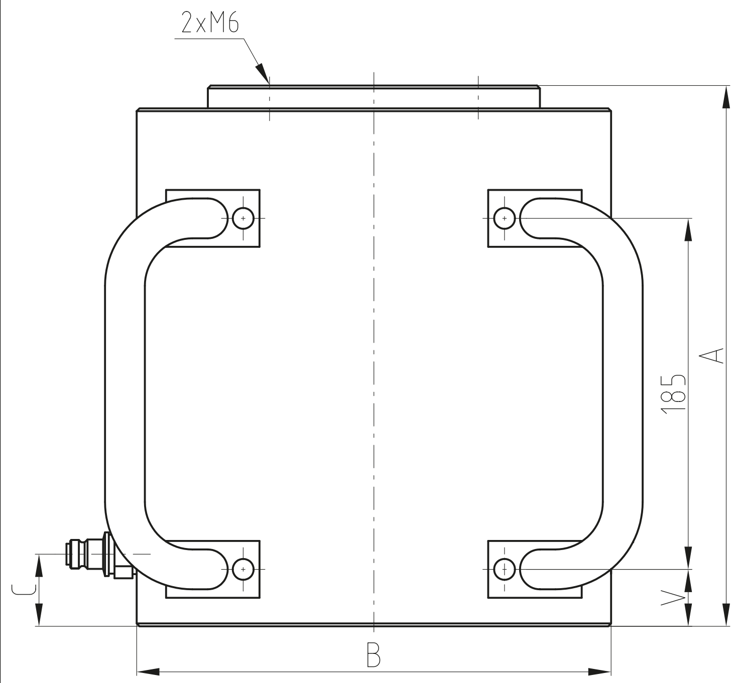
CX250B-100
